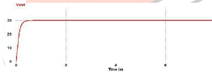
Figure 9: (d) Voltage Output of Boost Converter (Vout = 29.69v)
